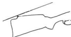
Monte Carlo tipas
